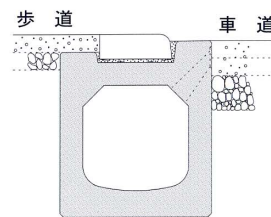
セミフラット乗り入れ H=20
